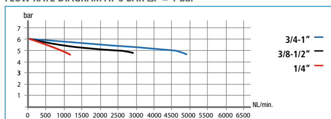
DIAGRAMMA DI PORTATA CON PRESSIONE A 6 BAR \Delta P = 1 bar FLOW RATE DIAGRAM AT 6 BAR \Delta P = 1 bar
