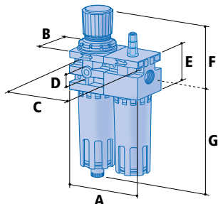
Scarico condensa manuale/semiautomatico Manual/semiautomatic condensate exhaust device
